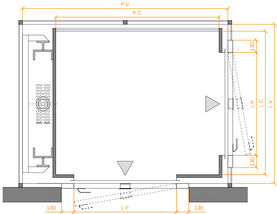
PIATTAFORMA ELEVATRICE OLEODINAMICA IN TAGLIA 2 : 1 ABITAZIONI - COMUNITA' - CENTRI SPORTIVI - RISTORANTI
