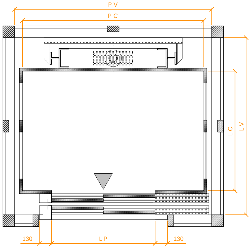
ASCENSORE OLEODINAMICO IN TAGLIA 2 : 1 - FOSSA RIDOTTA CENTRI COMMERCIALI - SUPERMERCATI
