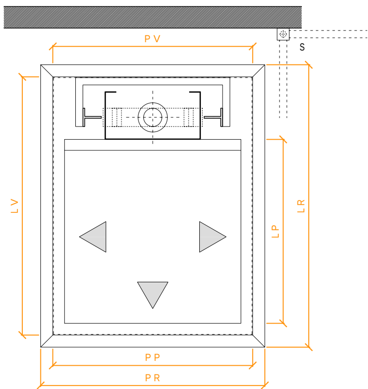
PEDANA DI SERVIZIO OLEODINAMICA - FERMATA A PAVIMENTO ABITAZIONI - COMUNITA' - HOTEL - RISTORANTI - BAR - OSPEDALI
