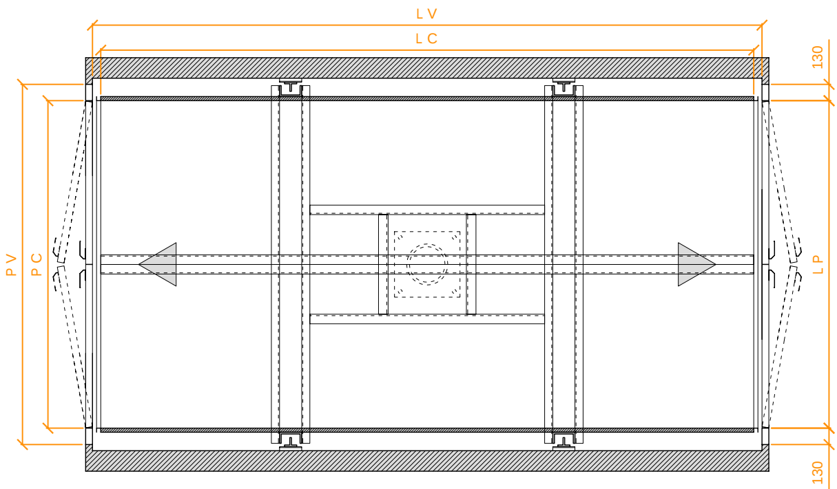
PEDANA ELEVATRICE MONTAUTO SENZA PERSONE A BORDO PISTONE TELESOPICO a 2 - 3 SFILAMENTI PARCHEGGI AUTO - GARAGE - UTENTI PRIVATI
