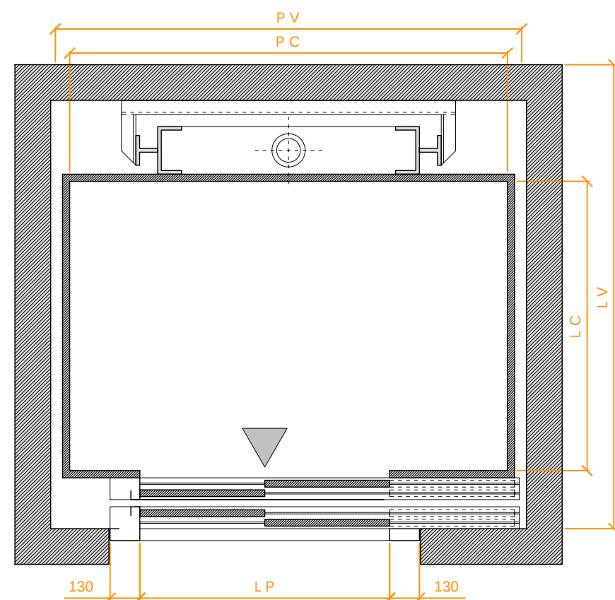
ASCENSORE OLEODINAMICO A SPINTA DIRETTA - VANO PROPRIO OSPEDALI - HOTEL - CENTRI COMMERCIALI
