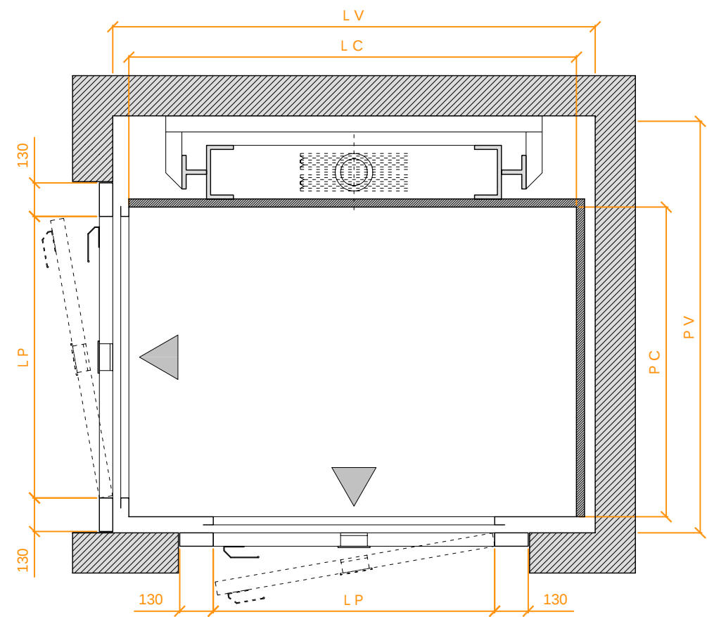
PIATTAFORMA ELEVATRICE OLEODINAMICA IN TAGLIA 2 : 1 ABITAZIONI - COMUNITA' - CENTRI SPORTIVI - RISTORANTI
